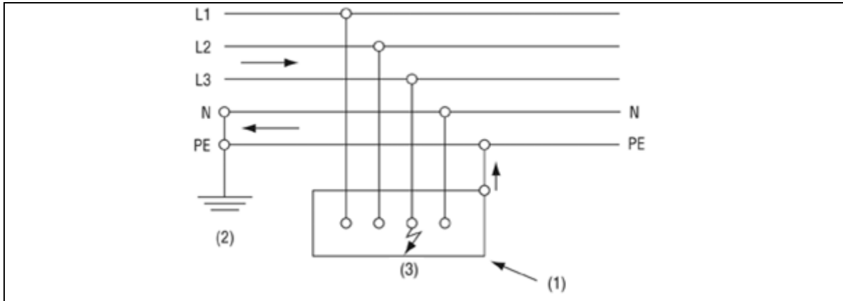
Figure 4.3. Boucle de défaut dans un schéma TN-S
