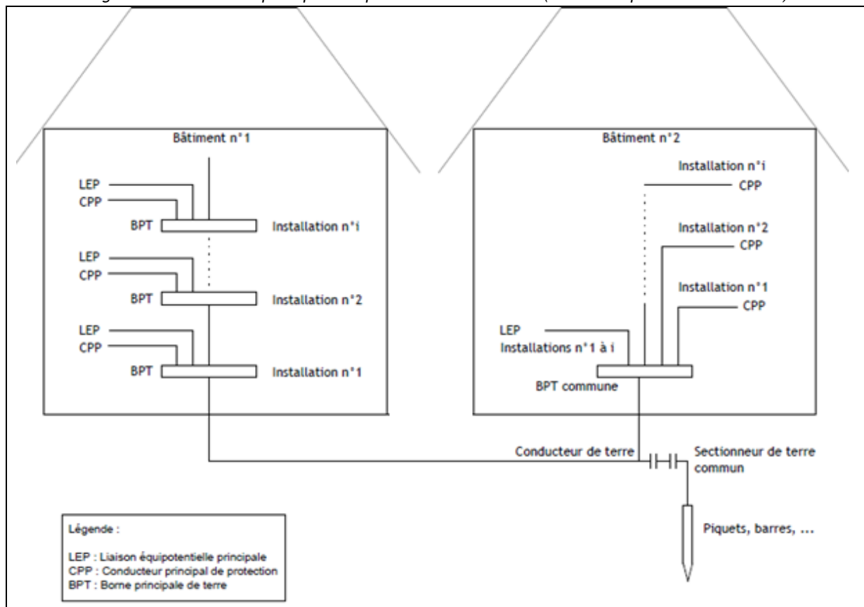
Figure 5.33. Schéma de principe de la prise de terre commune (cas visé au point c.1. 3 ème alinéa)
