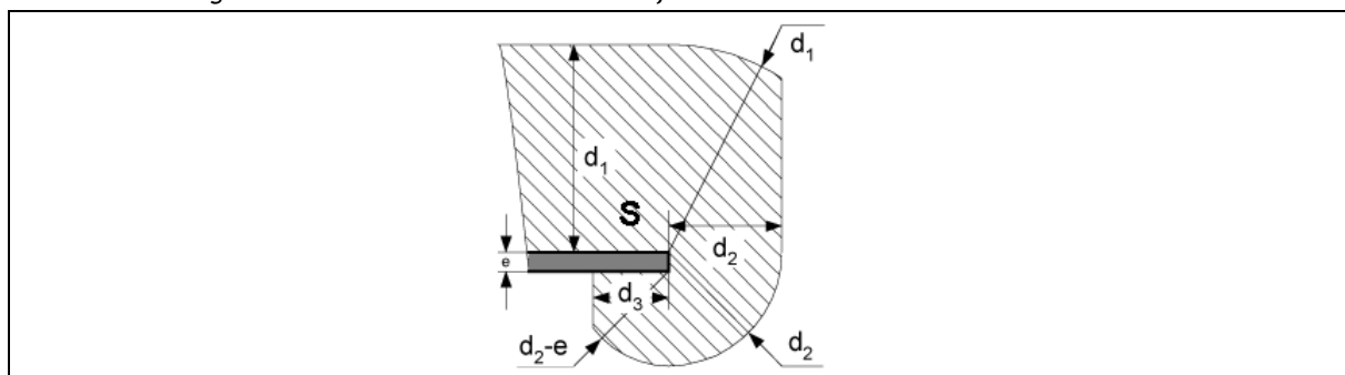
Figure 2.7. Volume d'accessibilité: la surface de circulation est limitée par un élément matériel
