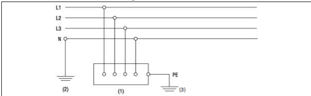
Figure 2.4. Schéma TT
