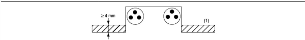
Figure 5.28. Coupe schématique d'une saignée
