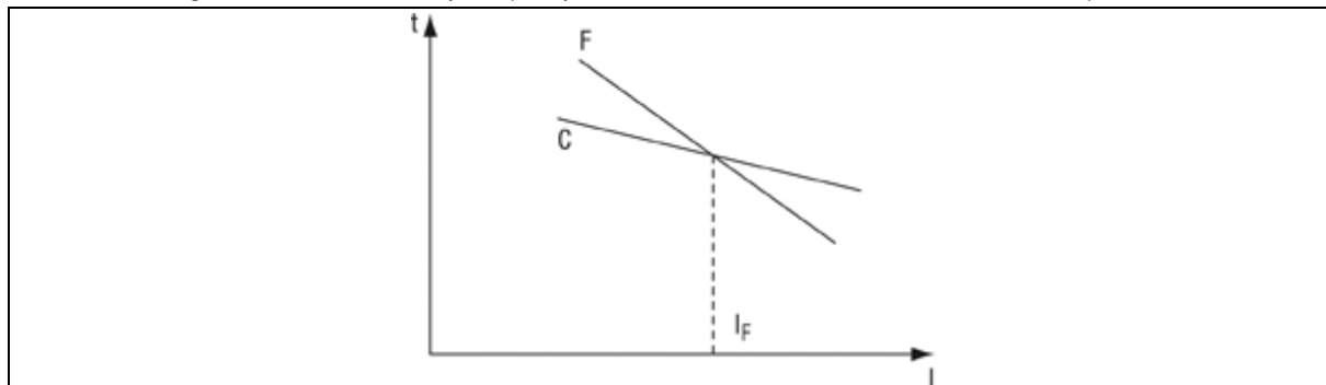
Figure 5.29. Choix du dispositif de protection contre les courts-circuits en cas de fusibles
