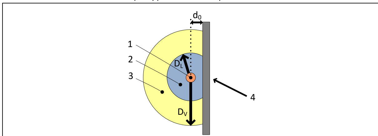
Figure 2.23. Représentation de la zone sous tension et de la zone de voisinage avec dispositif protecteur métallique mis à la terre
