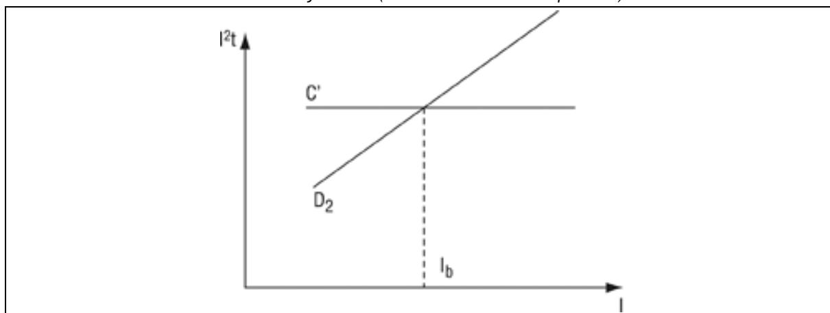
Figure 5.31. Choix du dispositif de protection contre les courts-circuits en cas de disjoncteurs (courant de court-circuit présumé)
